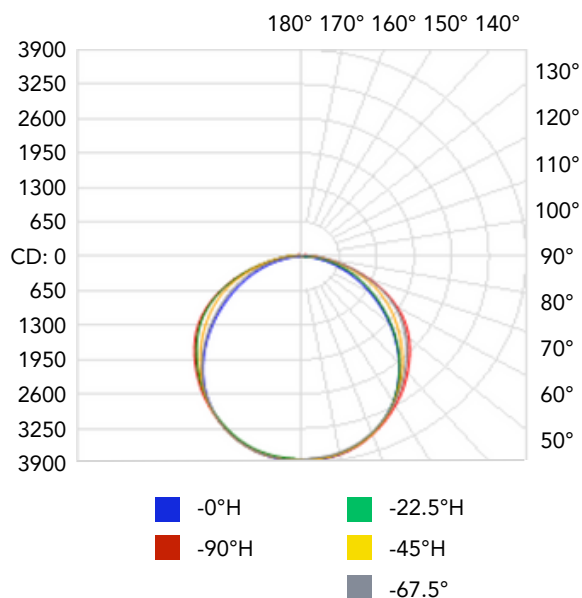
ISOFOOTCANDLE PLOT
